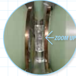
右) 振動試料型磁力計で実際に磁気テープの磁気を計測するところ。上部の黒い筒が振動を与える部分。上) 磁気テープは磁極間にセットされる。下) 詳しく説明してくれる今井社長。
